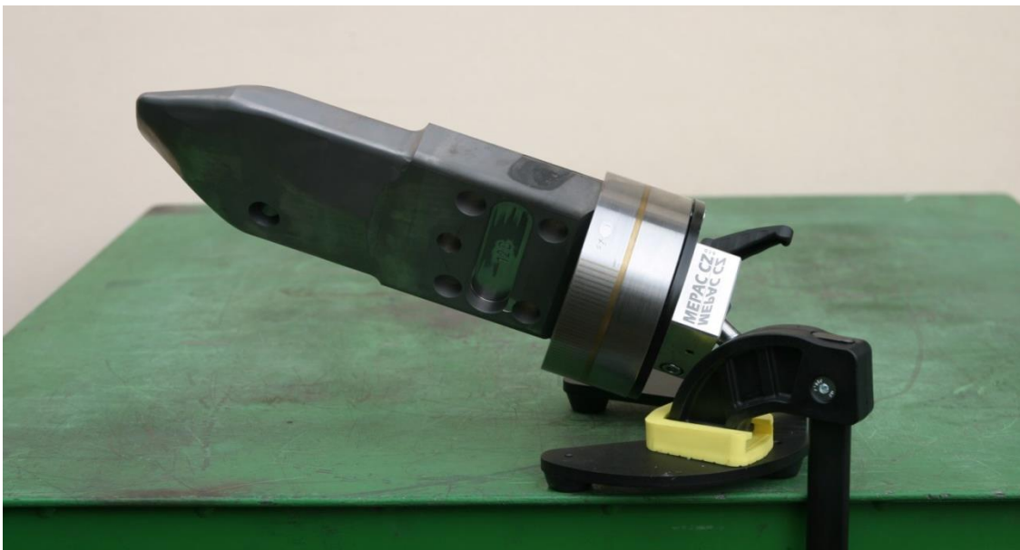
Ukázka uchycení tvarové vložky. S takto uchycenou vložkou je snadná manipulace při opracování díky polohovacímu magnetu. Hmotnost jazyku 3.5kg, rozměry – 30x900x225mm
