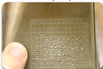
datumovník před opravou
